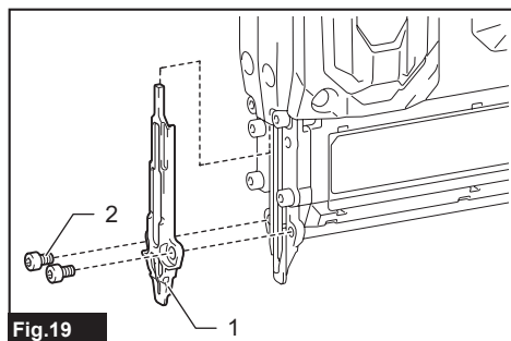
Fig.19 ► 1. Guía del impulsor 2. Perno de cabeza hexagonal
